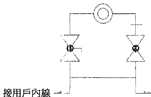
∅ 20m/m~40m/m 立式表位安裝組合參考示意圖
