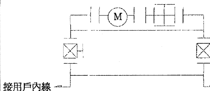
∅ 50m/m~100m/m 立式表位安裝組合參考示意圖
